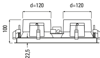
Seitenansicht
